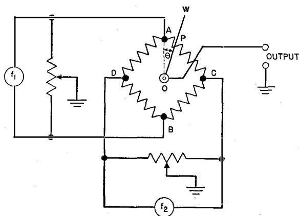
Fig. 4—Calibrator circuit.
